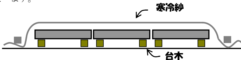
図 平床出芽の方法
